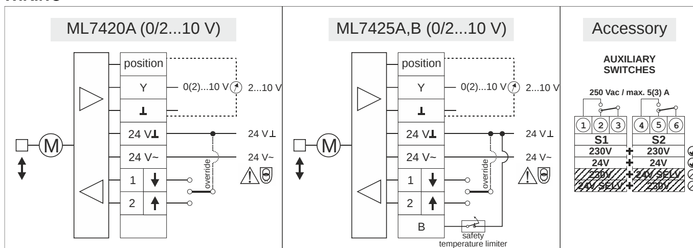
Fig. 3. Wiring
